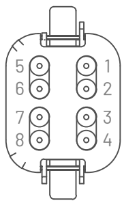
Anslutningskontakt DT06-08SA
