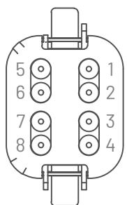
Anslutningskontakt DT06-08SA
