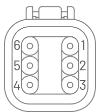
Anslutningskontakt DT06-06SA
