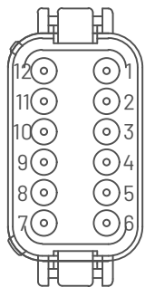
Anslutningskontakt DT06-12SA
